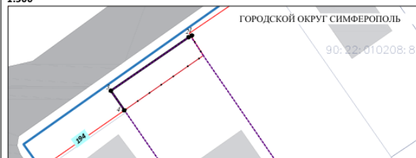
РАЗБИВОЧНЫЙ ЧЕРТЕЖ КРАСНЫХ ЛИНИЙ 1:500
