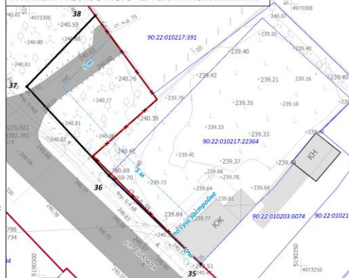
ФРАГМЕНТ РАЗБИВОЧНОГО ЧЕРТЕЖА КРАСНЫХ ЛИНИЙ
