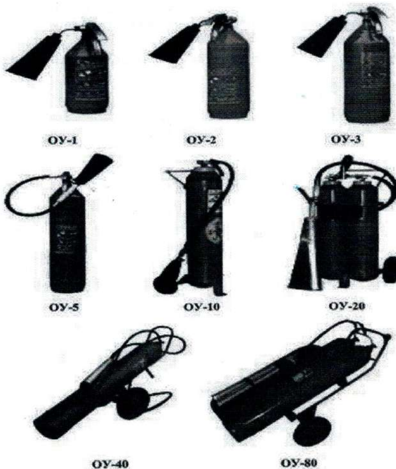
Технические характеристики углекислотных огнетушителей
