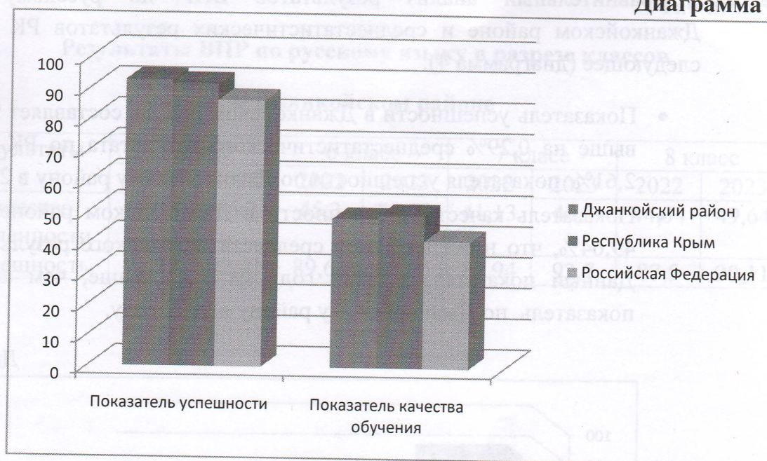
Диаграмма 3
