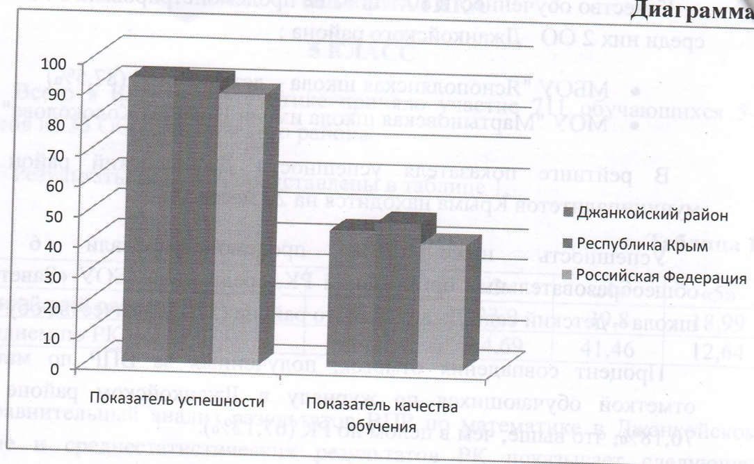
Диаграмма
