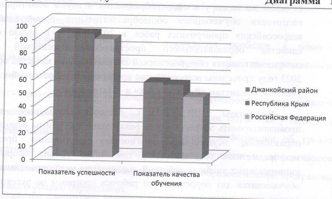
Диаграмма 1
