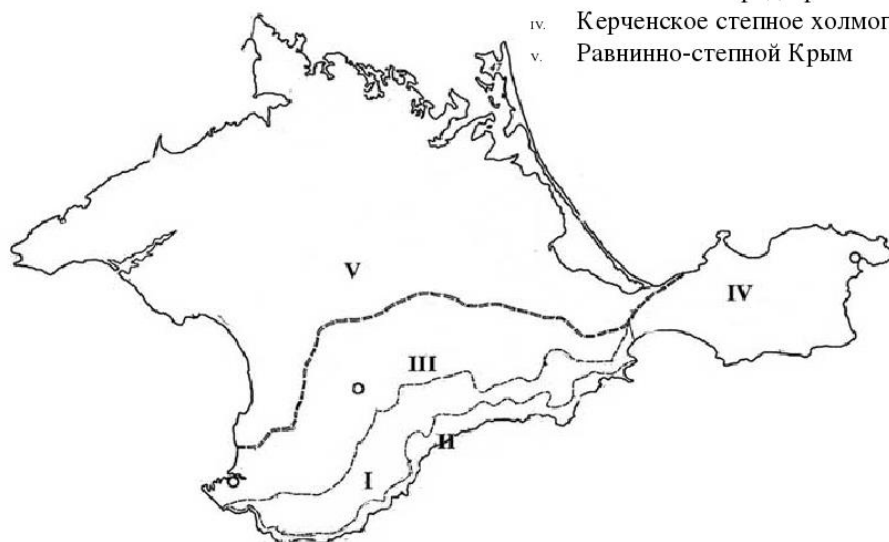
Физико-географическое районирование Крыма
