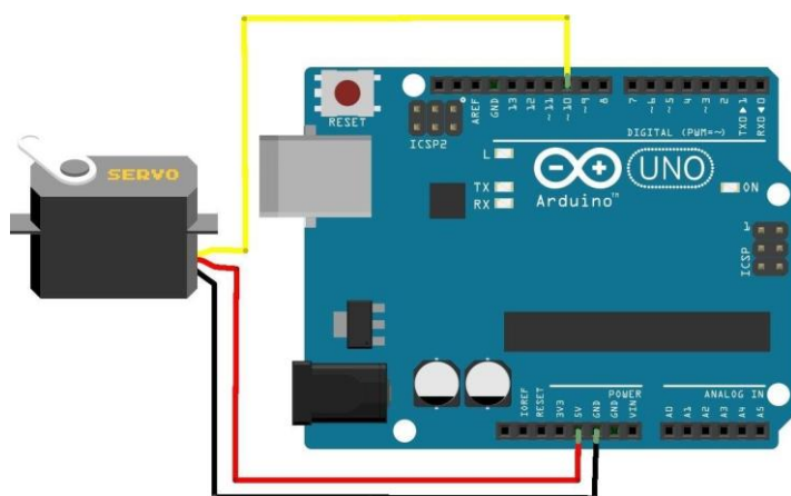
Схема подключения сервопривода на Arduino
