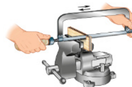
Рис. 5.27. Резание тонколистового металла
