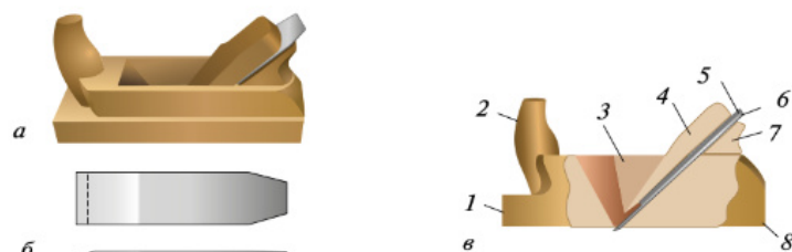
Рис. 4.2. Рубанок с деревянной колодкой: а — общий вид рубанка; б — железка (нож); в — основные части рубанка: 1 — колодка; 2 — передняя ручка-рожок; 3 — леток; 4 — деревянный клин; 5 — стружколом; 6 — нож; 7 — упор; 8 — подошва
