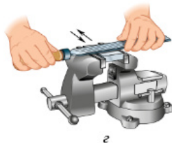
Рис. 5.36. Приёмы опилования: а — косым штрихом; б — поперечным штрихом; в — перекрёстным штрихом; г — продольным штрихом
