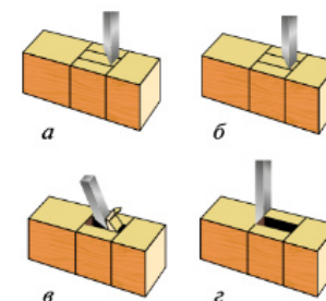
Рис. 4.56. Последовательность долбления гнезда
