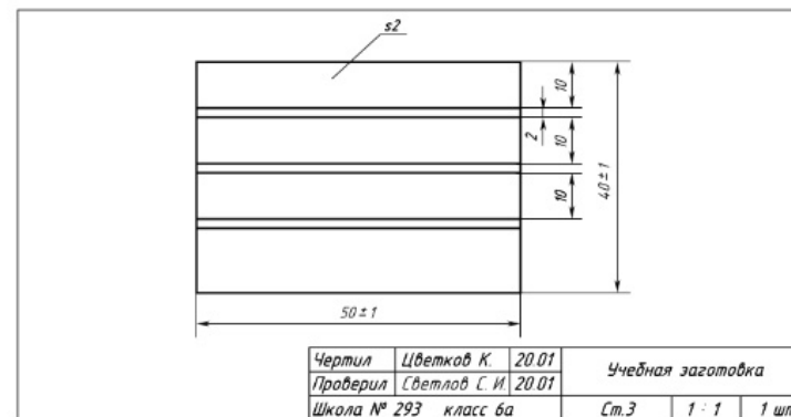
Рис. 5.22. Чертёж учебной заготовки для рубки полос
