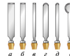
Рис. 4.24. Резцы-стамески: а, б, в — плоские; г, д — скруглённые; е — стамеска-крючок
