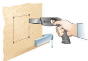
Рис. 4.44. Приём выпиливания внутреннего контура узкой выкружной ножовкой
