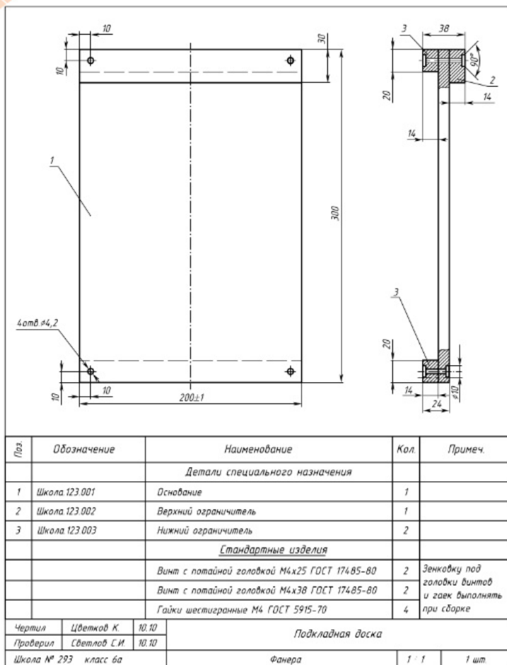
Рис. 1.7. Сборочный чертёж подкладной доски для столярного верстака
