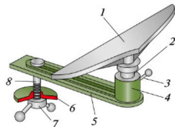
Рис. 4.8. Подручник: 1 — наклонное ложе; 2 — стержень; 3 — рукоятка; 4 — втулка с приливом; 5 — брус; 6 — прижим; 7 — гайка с рукояткой; 8 — болт
