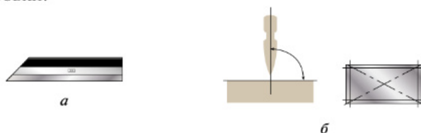
Рис. 5.37. Проверка лекальной линейкой: а — лекальная линейка; б — проверка опилённой поверхности на просвет
