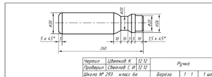
Рис. 4.40. Чертёж ручки резца-стамески
