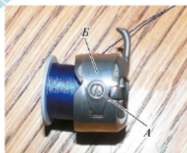
Рис. 6.14. Регулирование натяжения нити шпульного колпачка
