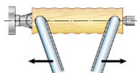
Рис. 4.33. Приёмы точения боковыми частями лезвия стамески
