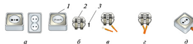
Рис. 11.8. Розетки электрические, их устройство и подключение: а — виды розеток; б — основные части розетки (1 — крышка; 2 — основание; 3 — крепёжный винт); в — подключение одного провода, оконцованного тычком, к основанию; г — подключение двух проводов к основанию розетки; д — розетка в собранном виде
