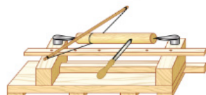
Рис. 4.3. Модель древнеегипетского станка с лучковым ручным приводом
