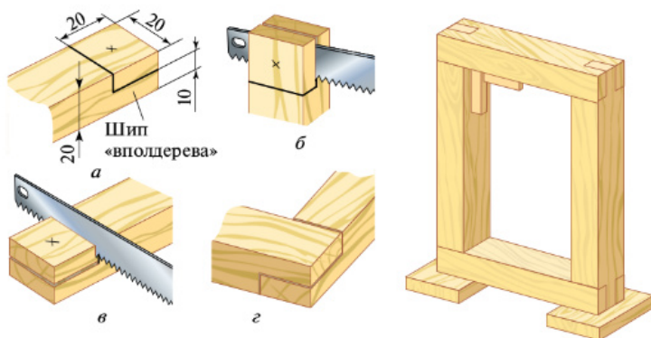
Рис. 4.58. Последовательность изготовления шипа «вполдерева»:
