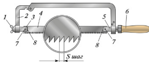
Рис. 5.24. Ручная слесарная ножовка с раздвижной рамкой
