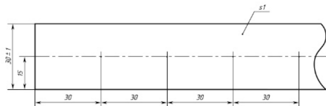
Рис. 5.54. Учебная заготовка для заклёпочного шва
