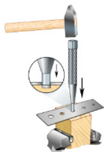
Рис. 5.48. Пробивание отверстий бородком
