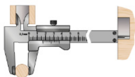
Рис. 4.14. Приёмы измерения древесины штангенциркулем
