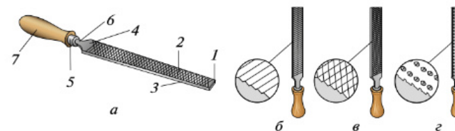
Рис. 5.31. Напильники: а — основные части:
