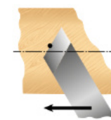
Рис. 4.34. Приём точения стамеской с косым срезом
