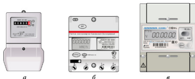
Рис. 11.11. Однофазные счётчики электрической энергии: а — одностарифный; б — двухтарифный; в — многотарифный
