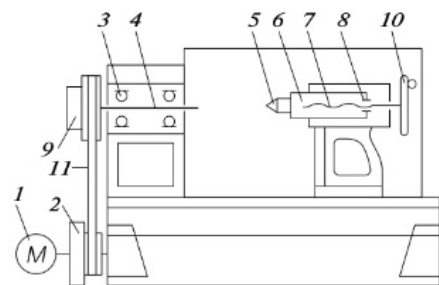
Рис. 3.6. Кинематическая схема токарного станка СТД-120М:
