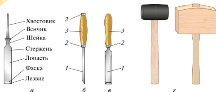
Рис. 4.53. Инструменты для долбления:
