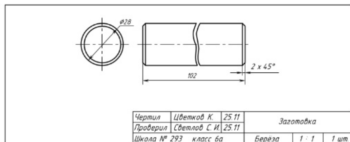
Рис. 4.39. Чертёж цилиндрической заготовки
