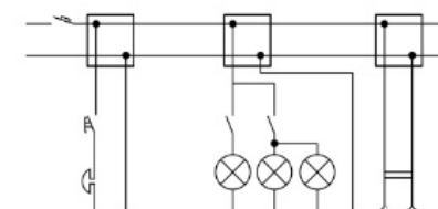
Рис. 11.13. Электрическая схема квартирной электропроводки
