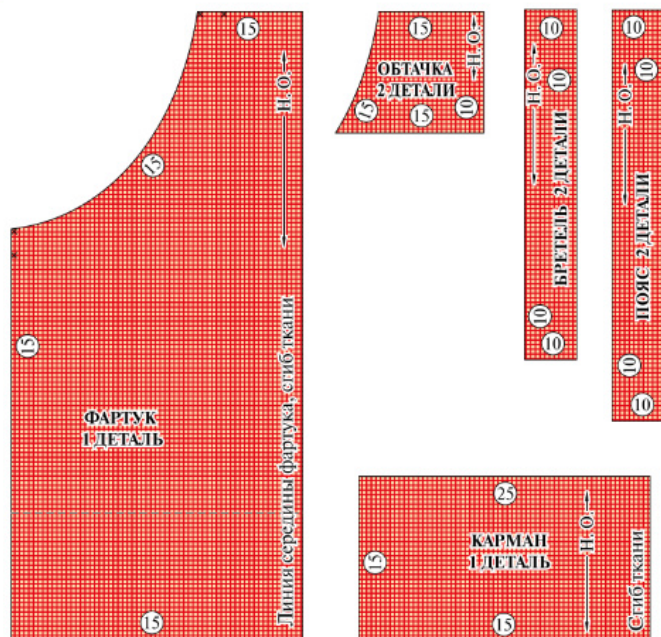
Рис. 6.29. Детали выкройки фартука
