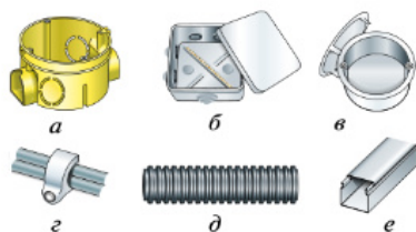
Рис. 11.10. Виды установочных изделий: а — коробка установочная; б — коробка ответвления; в — распаячная коробка; г — скоба для провода; д — труба гофрированная; е — короб пластмассовый (кабель-канал)
