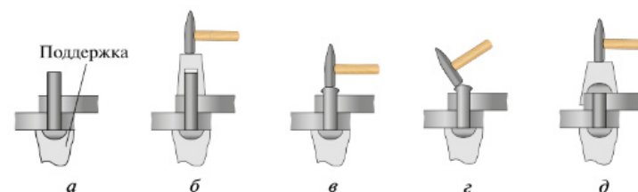
Рис. 5.47. Соединение деталей заклёпками с полукруглой головкой: а — установка заклёпки и поддержки в слесарных тисках; б — осаживание склёпываемых листов натяжкой; в — осаживание (расклёпывание) стержня; г — придание формы замыкающей головке; д — оформление замыкающей головки обжимкой
