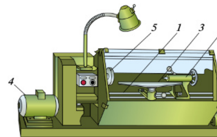
Рис. 4.9. Токарный станок для обработки древесины
