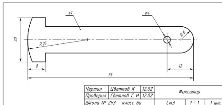
Рис. 5.40. Чертеж фиксатора
