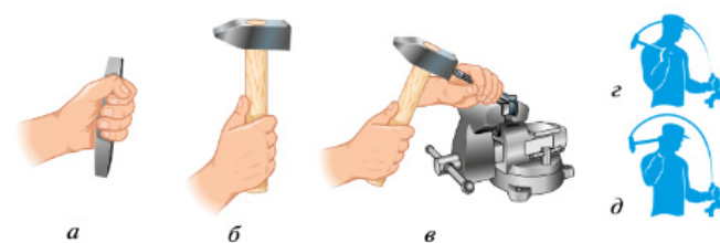
Рис. 5.19. Приёмы захвата инструмента и виды ударов молотком: а — приём захвата зубила; б — приём захвата молотка; в — кистевой удар; з — локтевой удар; д — плечевой удар
