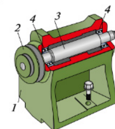
Рис. 4.6. Передняя бабка: 1 — корпус; 2 — двухступенчатый шкив; 3 — шпиндель; 4 — подшипники
