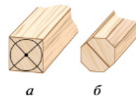
Рис. 4.25. Заготовка: а — разметка торцов; б — подготовленная заготовка
