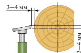
Рис. 4.31. Установка подручника
