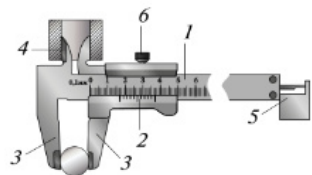
Рис. 5.12. Устройство штангенциркуля: 1 — штанга с миллиметровыми делениями; 2 — подвижная рамка с делениями (нониус); 3 — губки для измерения наружных размеров; 4 — губки для измерения внутренних размеров; 5 — глубиномер; 6 — фиксатор (фиксирующий винт)
