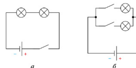
Рис. 11.12. Последовательное (а) и параллельное (б) включение ламп
