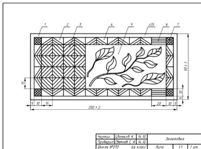
Рис. 8.7. Чертёж заготовки: 1 — контурное поле; 2 — орнаментальная полоса; 3 — резное поле из 16 квадратов 15 × 15 мм; 4 — свободные места на орнаментальной полосе; 5 — резное поле; 6 — прямоугольник; 7 — квадрат 10 × 10 мм
