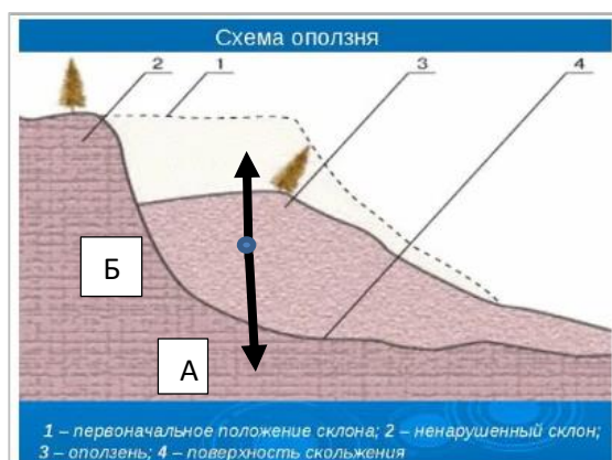
Рис. 2. Схема оползня
