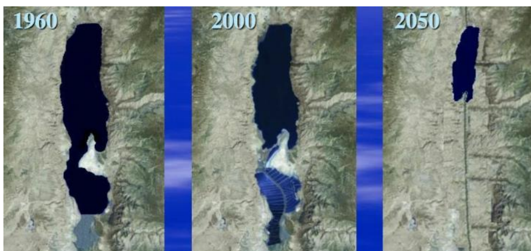
Рис. 3. Изменение уровня воды Мёртвого моря
