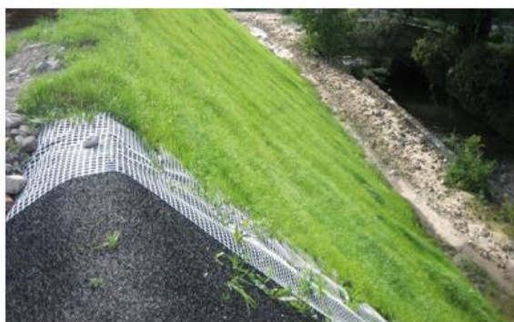
Рис. 7. Укрепление склона травянистой дернообразующей растительностью
