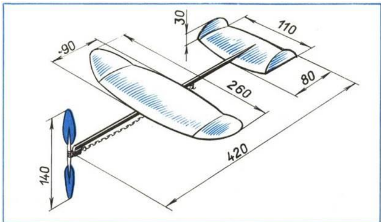
Модели самолетов
