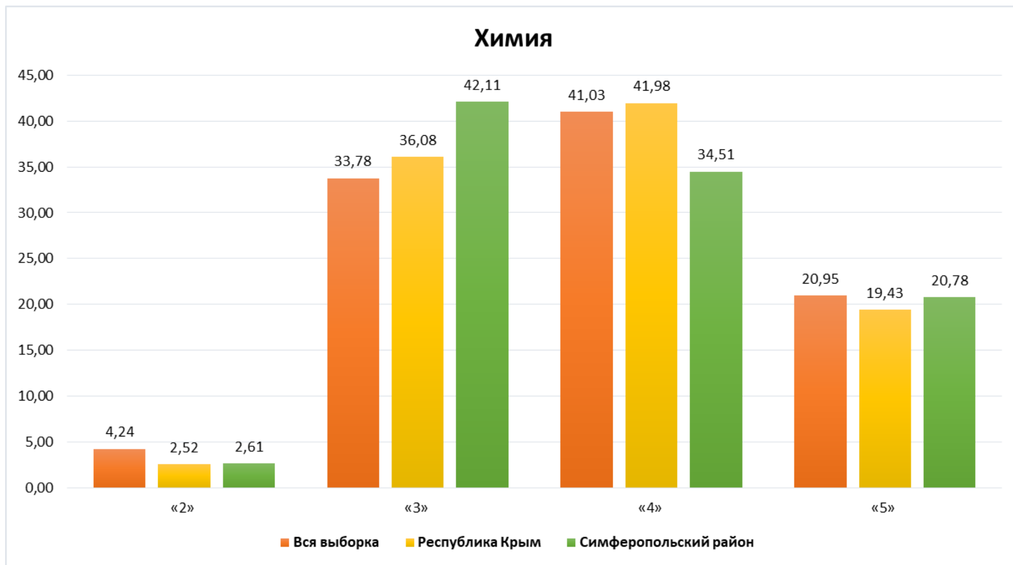
Диаграмма 10 «Химия»
