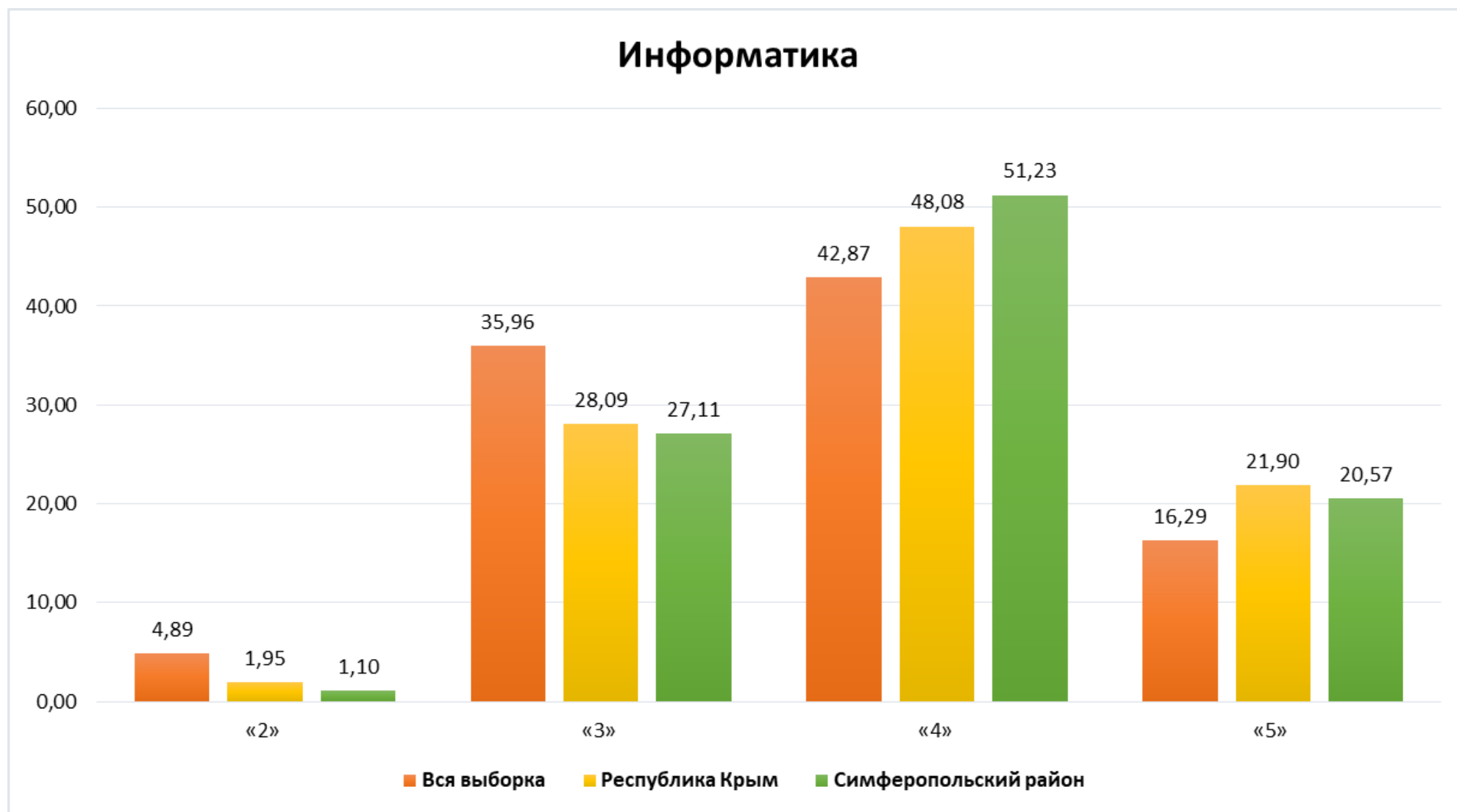
Диаграмма 11 «Информатика»
