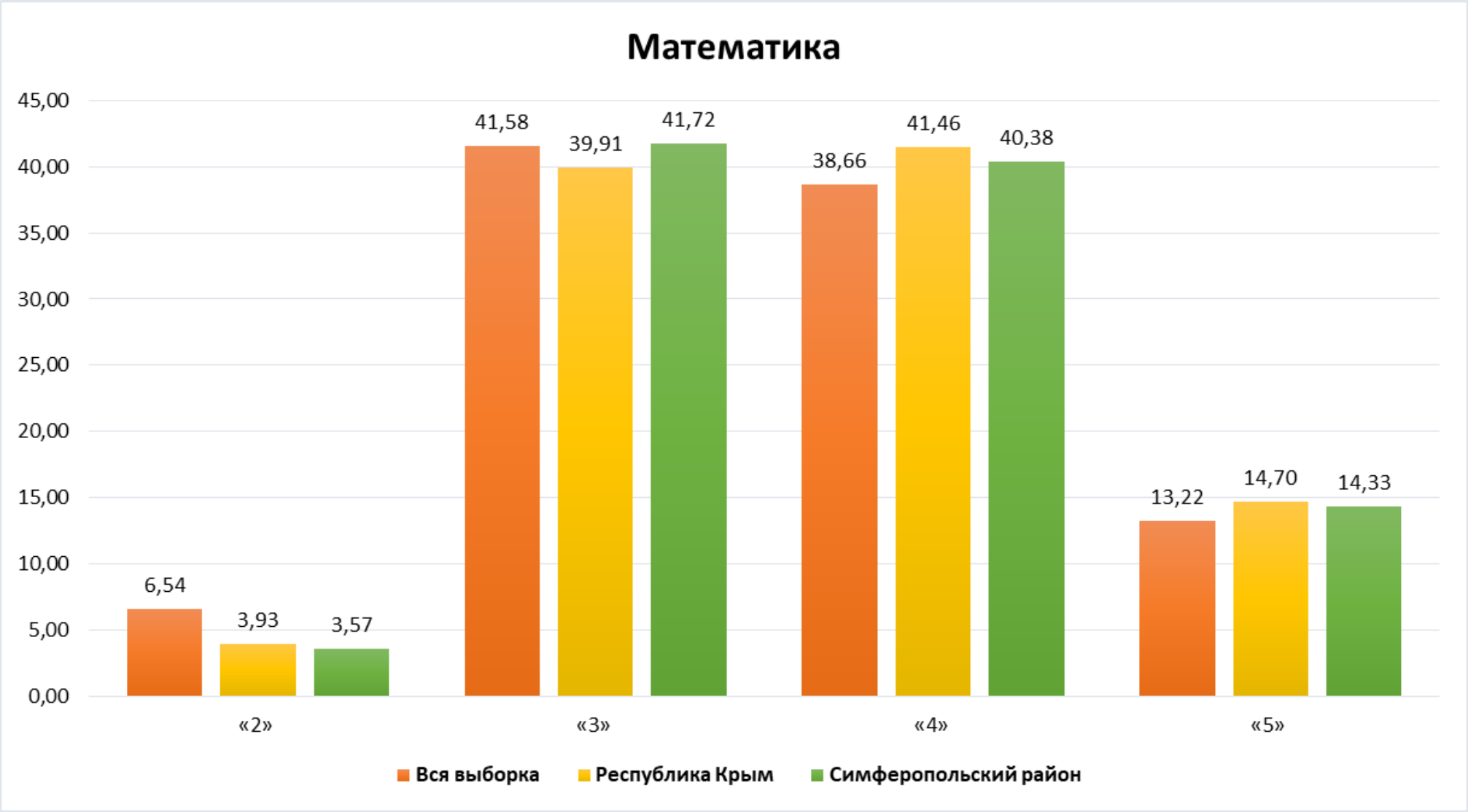
Диаграмма 2 «Математика»
