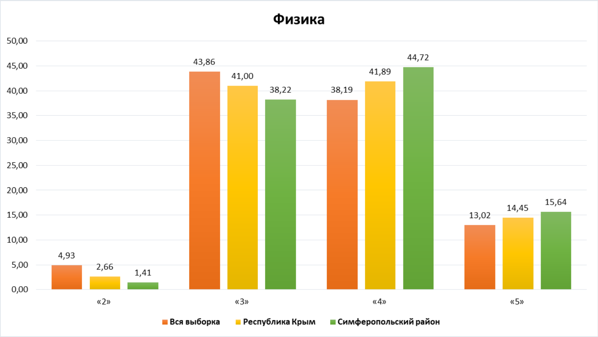
Диаграмма 8 «Физика»
