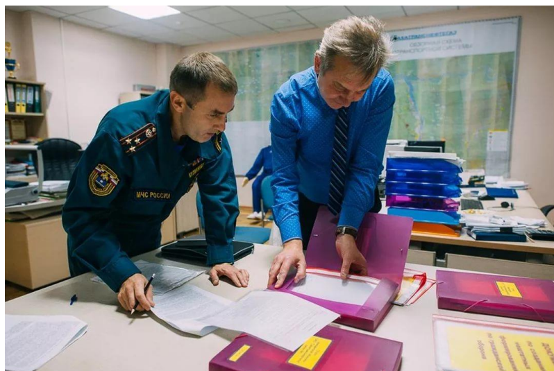
Документарная проверка
