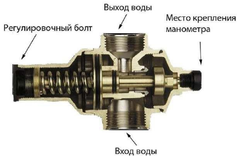
Регулятор расхода и давления воды.
